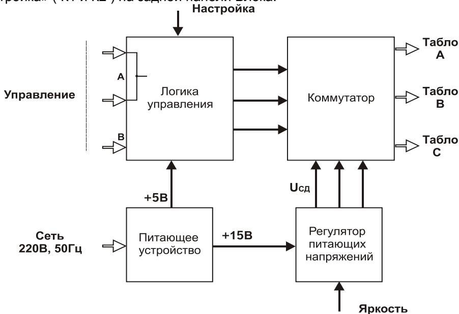
Рисунок 2.1 - Структурная схема блока TP-141
