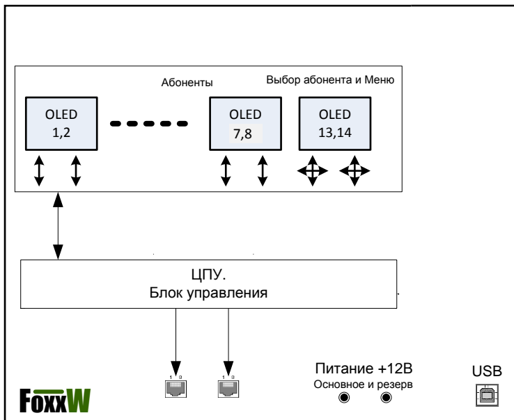
Рисунок 2.1 - Блок TP-813. Структурная схема
