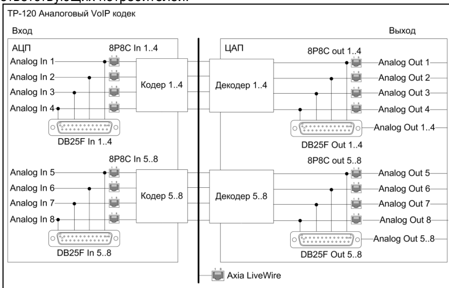
Рисунок 4.1- Схема функциональная
