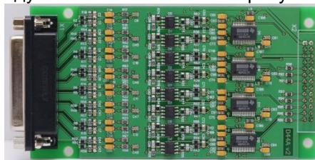
Рисунок 2.4 - Модуль TP-122-1
