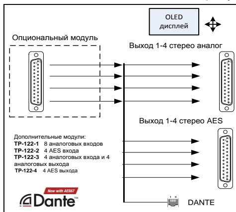
Рисунок 2.1 - Блок TP-122, Схема функциональная
