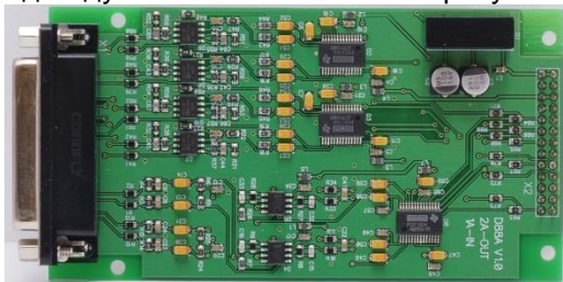
Рисунок 2.6 - Модуль TP-122-3
