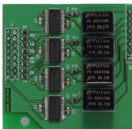
Рисунок 2.7 - Модуль TP-122-4
