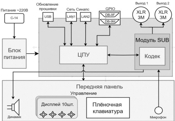
Рисунок 2.1 - Блок TP-832. Структурная схема
