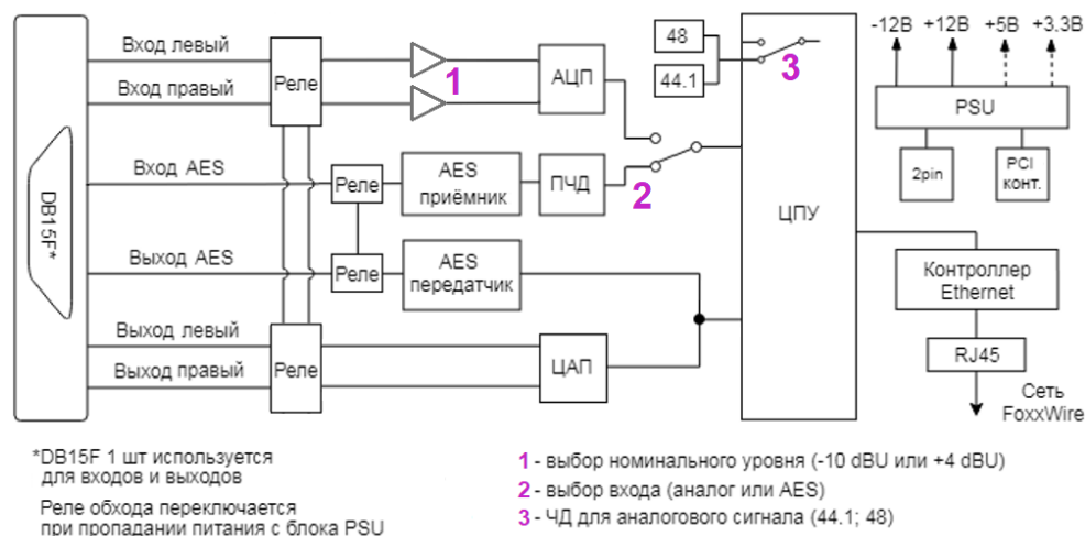
Рисунок 2.1 - Плата TP-322к, Схема структурная
