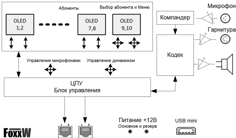
Рисунок 2.1 - Блок TP-808. Структурная схема
