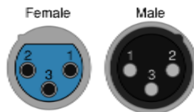
Рисунок 2.5 - Разъемы XLR F и XLR M
