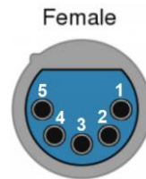
Рисунок 2.7 - Цоколёвка разъёма XLR5 F
