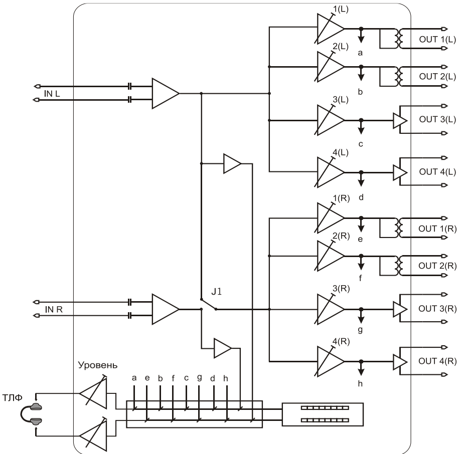
Рисунок 1 - TP-103М (TP-103М-1). Схема структурная
