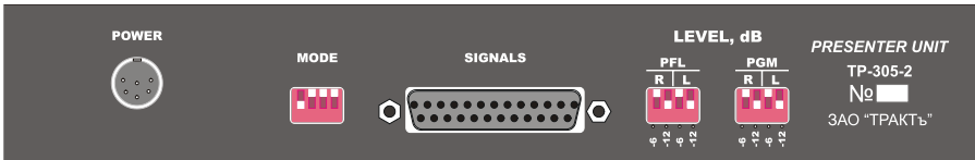
Рис.2. Задняя панель блока ведущего TP-305-2.
