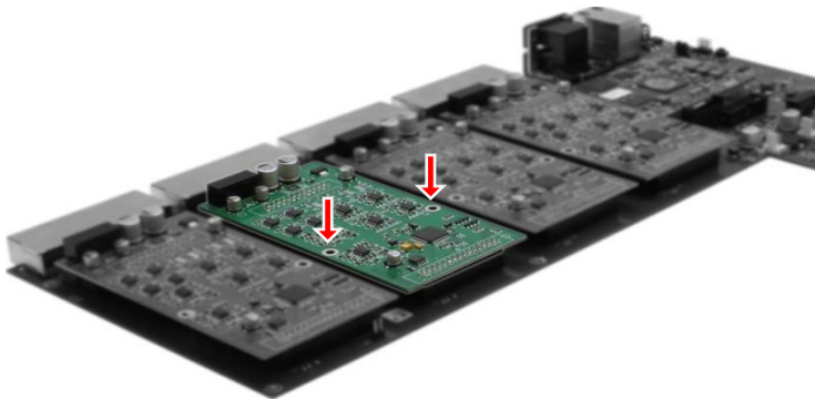
Рисунок 2.6 – Установка модуля TP-804-Analog
