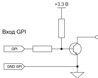
Рисунок 2.12 - Вход GPI, схема принципиальная.
