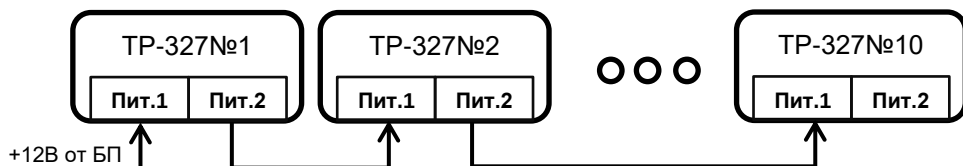
Рисунок 2.9 – Питание нескольких TP-327 от одного БП
