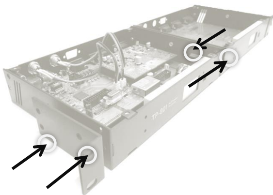
Рисунок 3.5 - Установка двух Блоков в стойку RACK 19”
