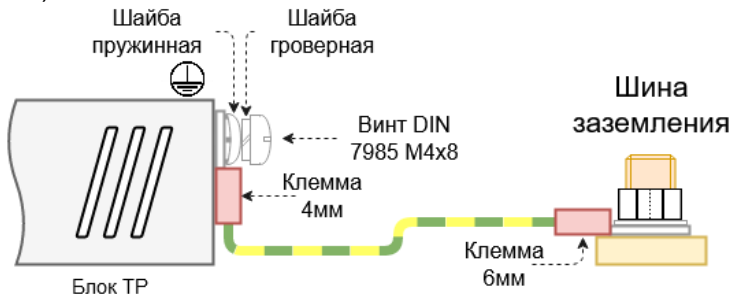
Рисунок 3.5 - Монтаж кабеля заземления
