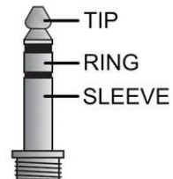
Рисунок 2.9 - Цоколёвка разъёма Jack 3.5mm TRS, 3pin
