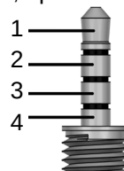
Рисунок 2.8 - Цоколёвка разъёма Jack 3.5mm TRRS, 4pin
