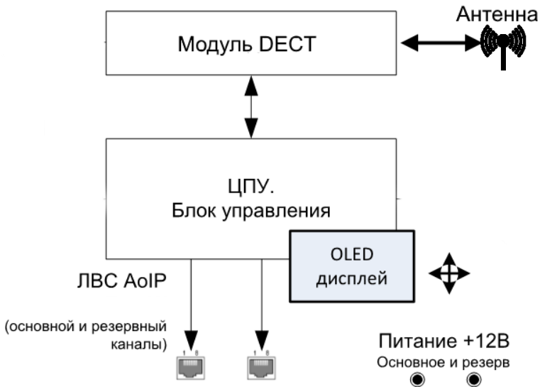
Рисунок 2.2 - TP-805. Схема структурная
