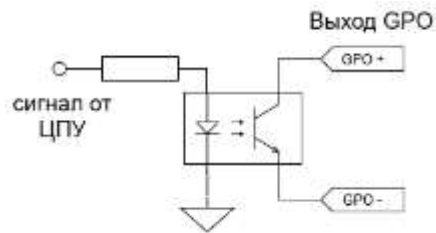
Рисунок 2.5 - Выход GPO,
