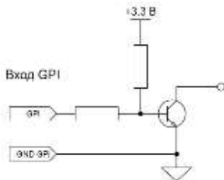
Рисунок 2.4 - Вход GPI,
