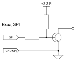
Рисунок 2.3 - Вход GPI, схема принципиальная.
