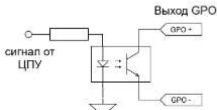
Рисунок 2.5 - Выход GPO, схема принципиальная.
