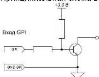
Рисунок 2.4 - Вход GPI, схема принципиальная.
