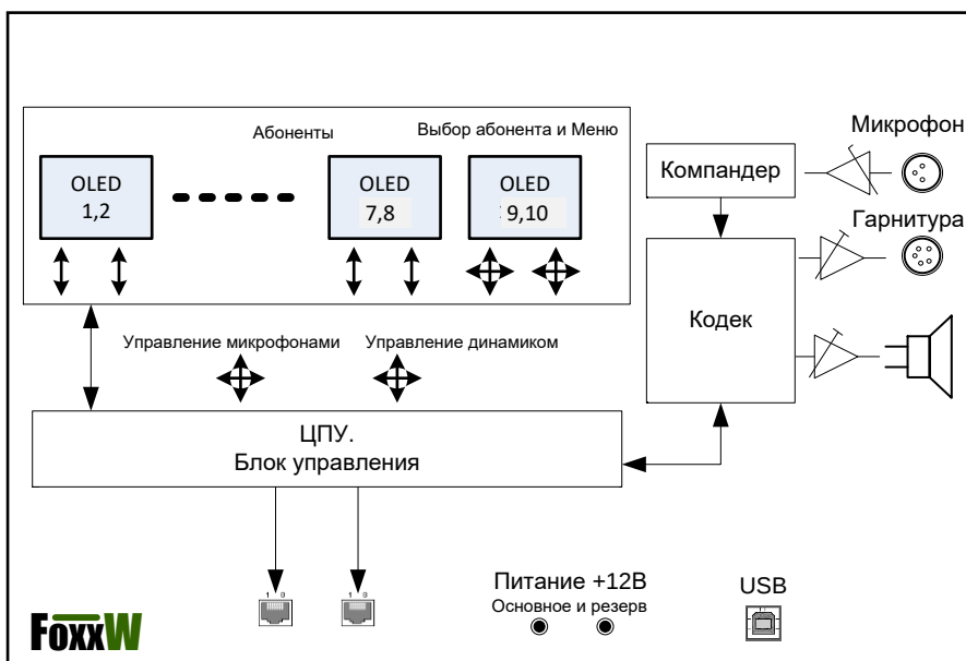
Рисунок 2.1 - Блок TP-808. Структурная схема
