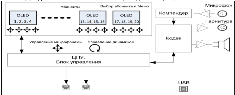
Рисунок 2.1 - Блок TP-820. Структурная схема
