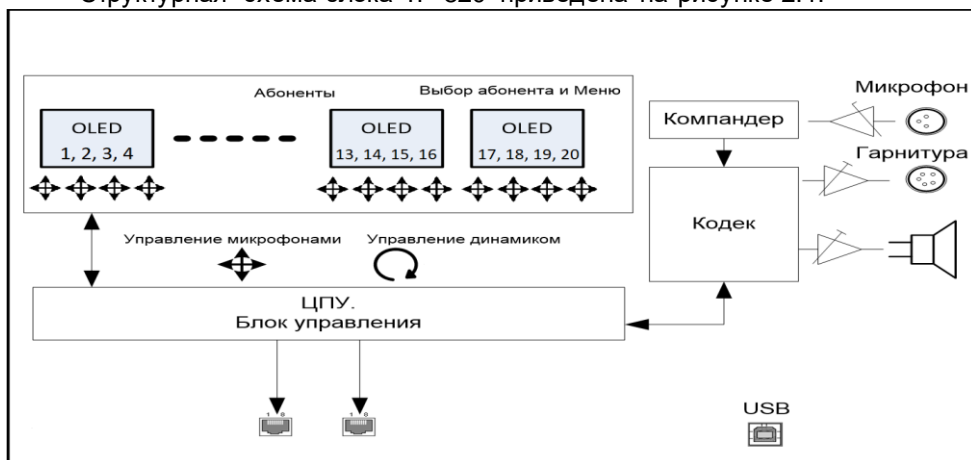
Рисунок 2.1 - Блок TP-820. Структурная схема
