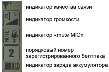
Рисунок 3.3 - Дисплей Белтпака
