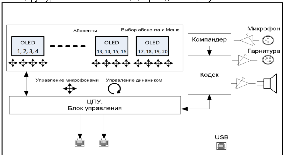
Рисунок 2.1 - Блок TP-820. Структурная схема
