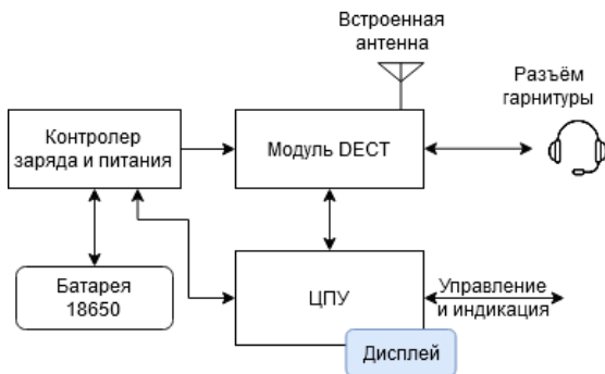
Рисунок 2.2 - TP-806. Схема структурная
