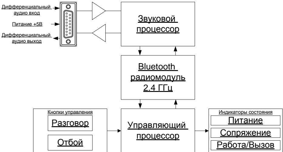
Рисунок 1.2 - Структурная схема TP-321
