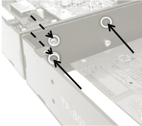
Рисунок 3.4 - Соединение двух Блоков
