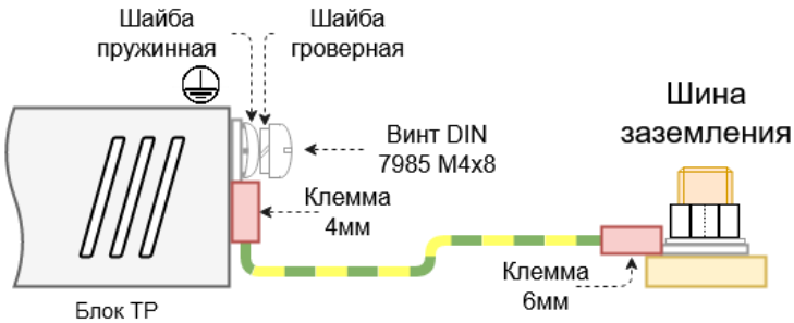
Рисунок 3.5 Монтаж кабеля заземления
