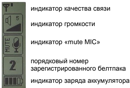
Рисунок 3.1 - Дисплей Белтпака
