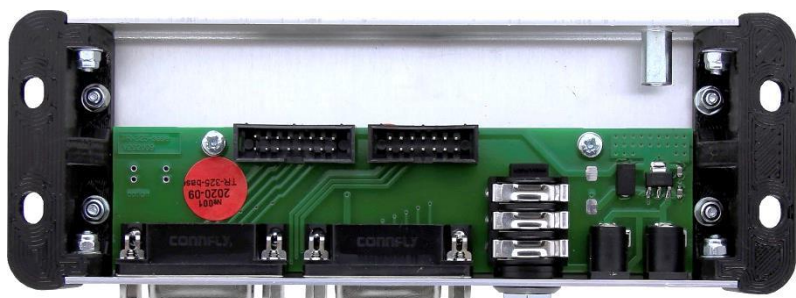
Рисунок 2.4 – Корпус TP-325, вид изнутри.
