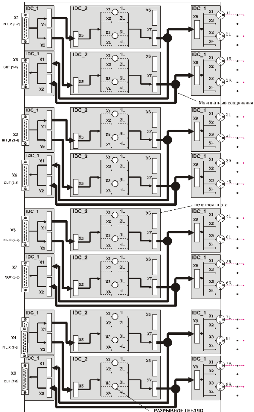
Рисунок 2.1 - Структурная схема
