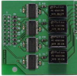
Рисунок 2.7 - Модуль TP-122-4, 4 AES выхода
