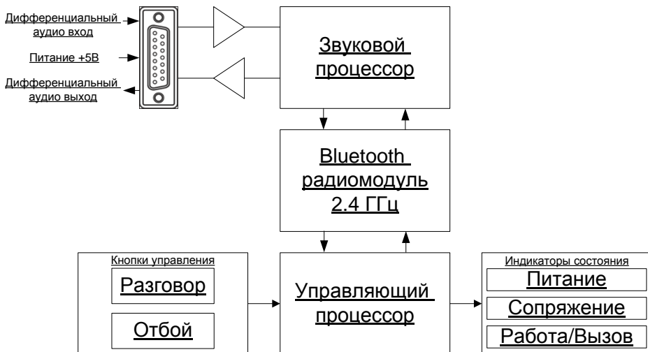
Рисунок 1.2 - Структурная схема TP-321
