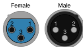
Рисунок 2.5 - Разъёмы XLR F и XLR M
