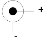
Рисунок 2.4 - Цоколёвка разъёма RCA
