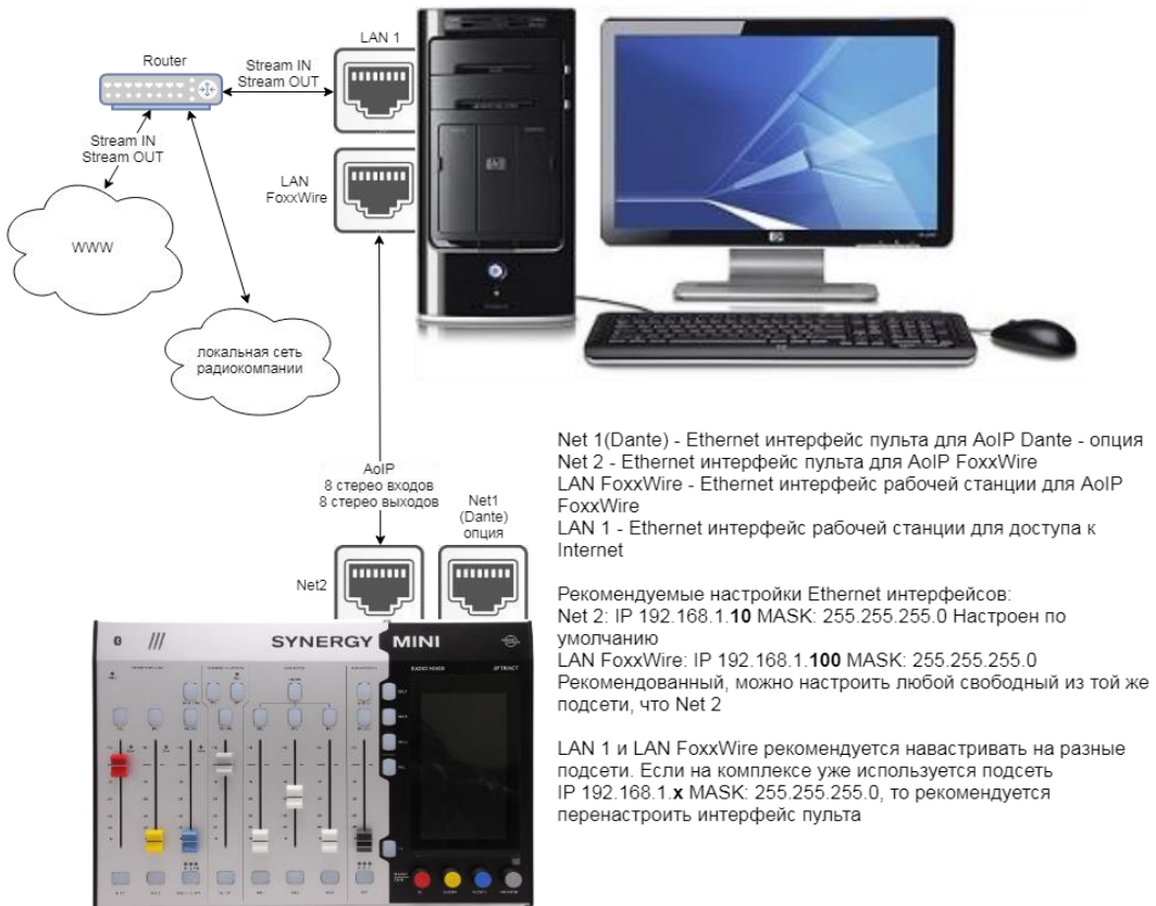
Рисунок 3.1 - Настройки сетевых интерфейсов
